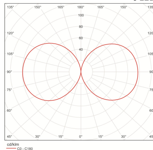
Curva de distribución SAL DECO-3 LED
