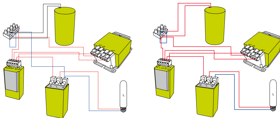
Cableado para sistema temporizado
